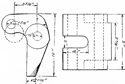
Fig. 2078. Plan. Fig. 2079. End Elevation.
